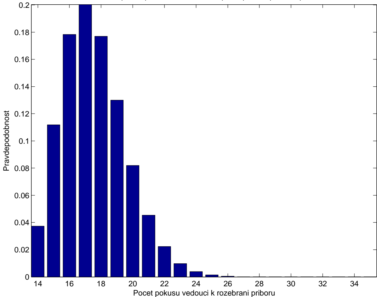
Rozdeleni pravdepodobnosti celkoveho poctu pokusu pro N=7 pristoru
