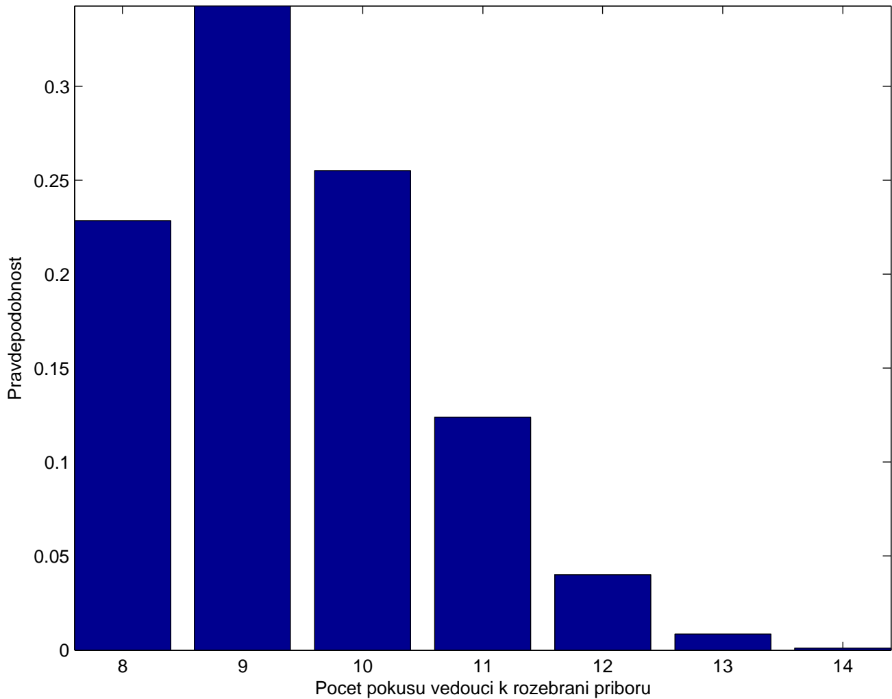
Rozdeleni pravdepodobnosti celkoveho poctu pokusu pro N=4 prбору
